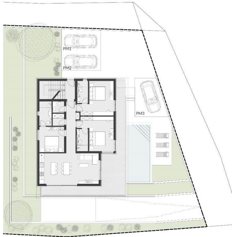
PRIZEMLJE
